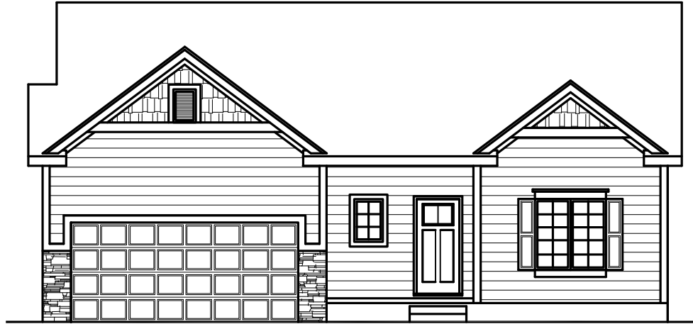
ELEV B
